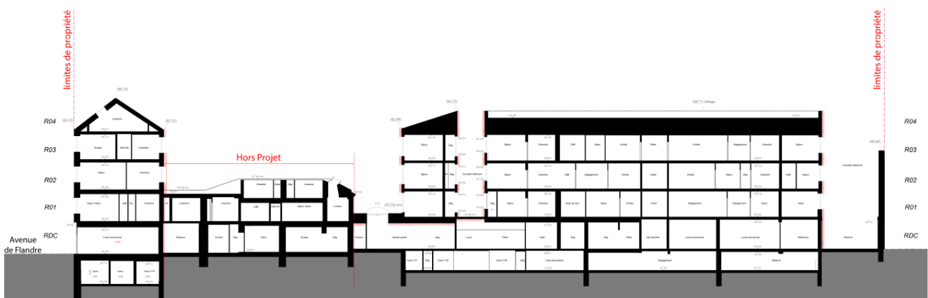
Coupe verticale état existant
